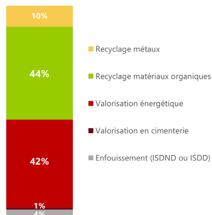
MODES DE TRAITEMENT EN PAYS DE LA LOIRE
