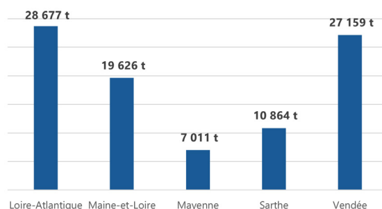
RÉPARTITION PAR ORIGINE GEOGRAPHIQUE
