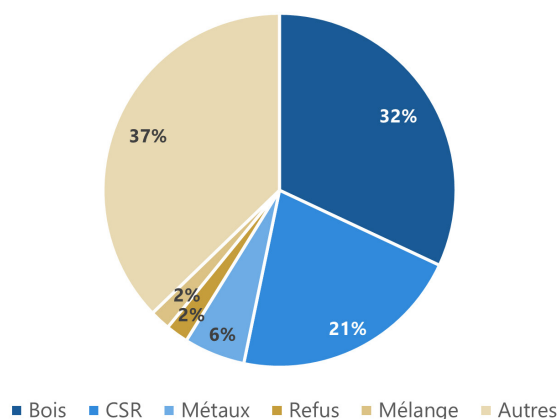
TYPE DE MATÉRIAUX TRAITÉS EN PAYS DE LA LOIRE
