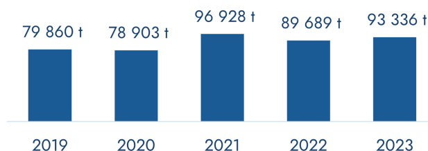
Tonnages collectés en Pays de la Loire
